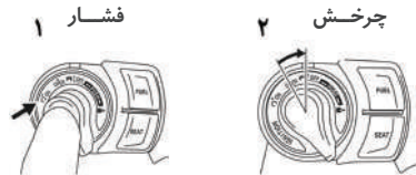
کلید FUEL ۱
