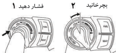
فشار دهید ۱
