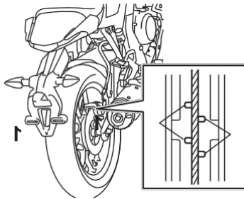
1. شیار نشانگر سایش لنت ترمز
