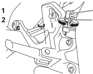
1. آر 2. مهره تنظیم سوئیچ چراغ ترمز عقب
