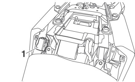
۱. جعبه فیوز
